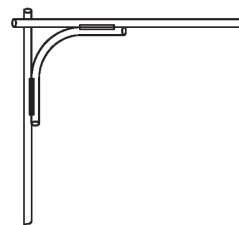
نحوه جوشکاری میلگردها در یک گوشه
